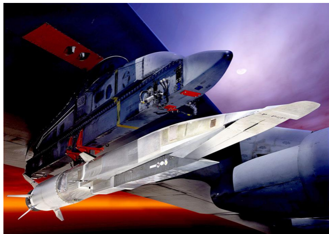
Х-51А Waverider под крылом бомбардировщика В-52
