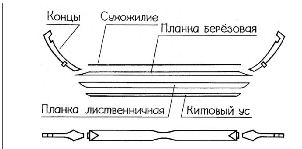
Детали восточносибирского (корякского) лука с мыса Тайгонос. Воспроизведено по: Глинский 1987: Рис. 3
