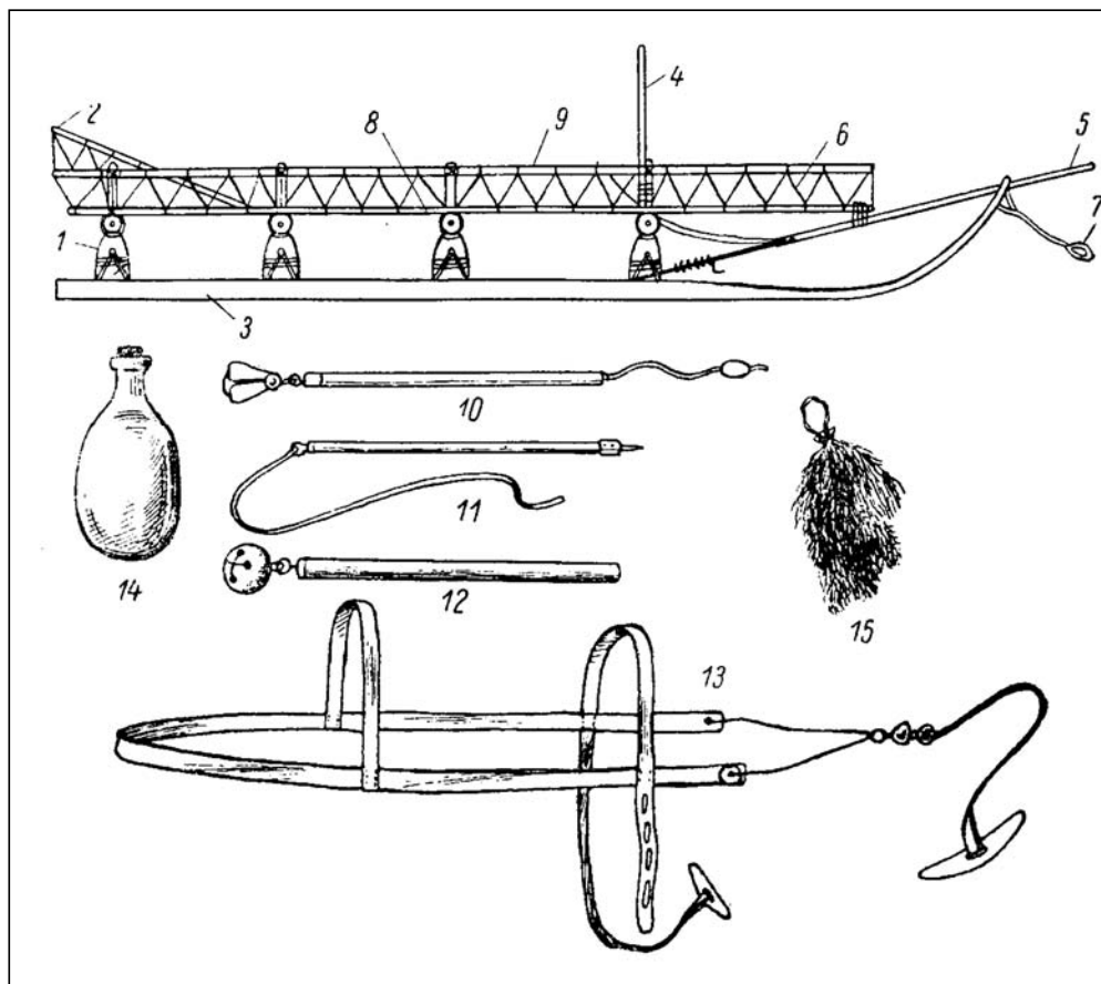
Детали эскимосской нарты, запрягаемой собаками (втор. четв. XX в.): 1 — копылье; 2 — задняя дуга; 3 — полоз; 4 — средняя дуга для держания; 5 — передняя дуга; 6 — ременная обвязка; 7 — петля для прикрепления тягового ремня; 8 — доска-сиденье; 9 — «нахлестка»; 10 — кнут с погремушками; 11 — остол; 12 — погремушка; 13 — упряжь, надеваемая на собаку; 14 — фляга для воды, чтобы смачивать полозья; 15 — кусок шкуры белого медведя, которым смачивают полозья. Воспроизведено по: Рубцова 1954: 540, рис. 39
