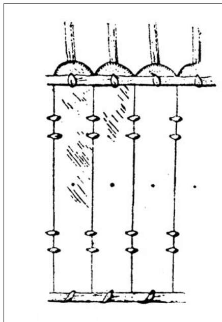
Крепление чукотского ламелярного доспеха (с внешней стороны). Воспроизведено по: Богораз 1991: 98, рис. 86b
