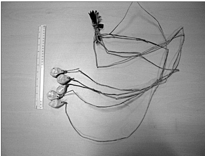
Пятихвостовая бола. Музейный центр «Наследие Чукотки» (МЦНЧ-2236)
