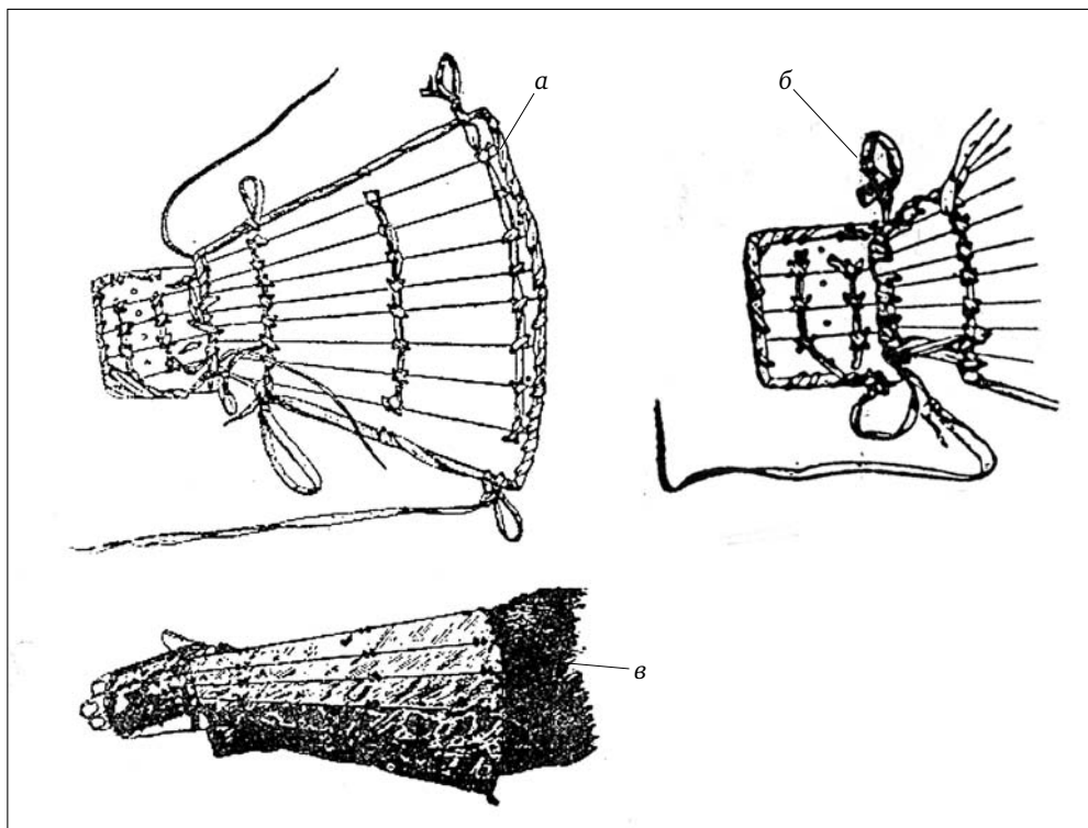
Железный наруч с лопастью для защиты верха кисти руки: а — вид изнутри; б — подробный вид крепления лопасти к наручу изнутри; в — наруч, надетый на руку воина. Воспроизведено по: Богораз 1991: 100, рис. 91а, б, с
