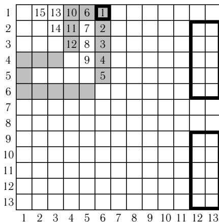
Рис. 19. Для клетки 1 жирными линиями выделена зона асимметрии. Серым цветом отмечены клетки верхнего левого угла 6 \times 6 , меняющие свой цвет
