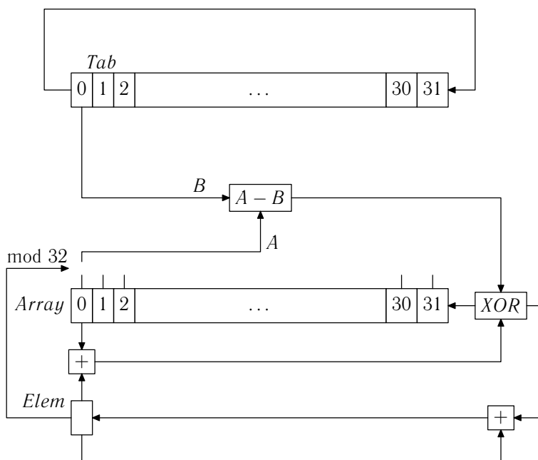
Рис. 1. Схема криптографического преобразования, используемого ОС Novell NetWare
