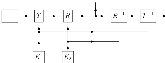
Рис. 3. Произведение двух систем S = RT
