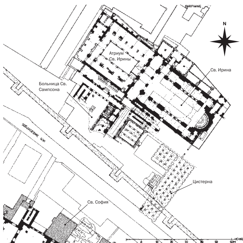
Св. Ирина с атриумом, цистерной (закрытой теперь) и остатками больницы Св. Сампсона
