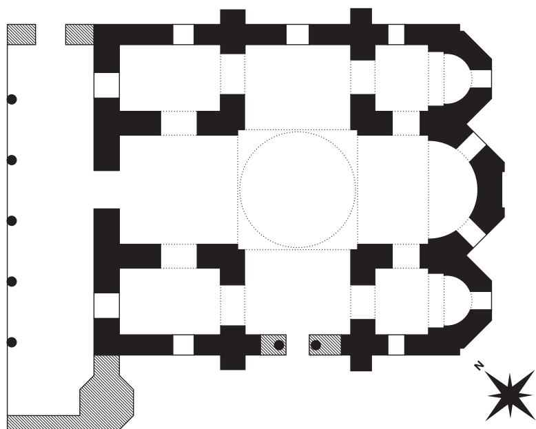
План церкви Atik Mustafa Paşa
