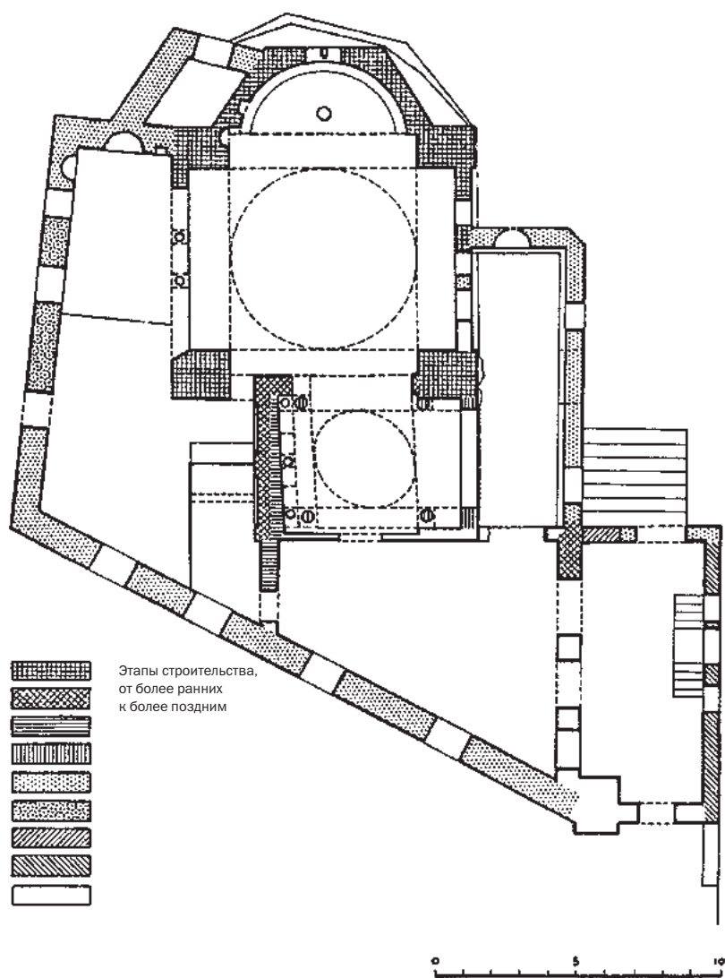
План Архангельской церкви
