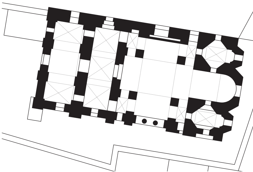
План Эски-Имарет (Христа Непостижимого?)
