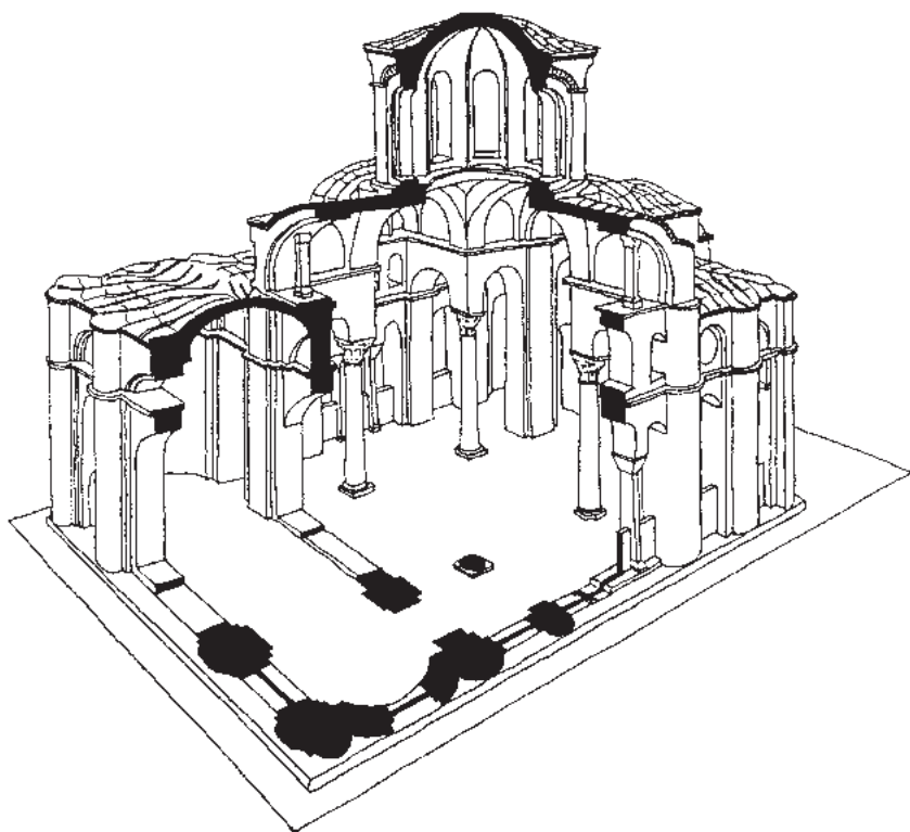
Мирелейон в разрезе
