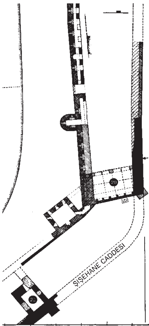
План дворца Багрянородного и конец Феодосиевой стены
