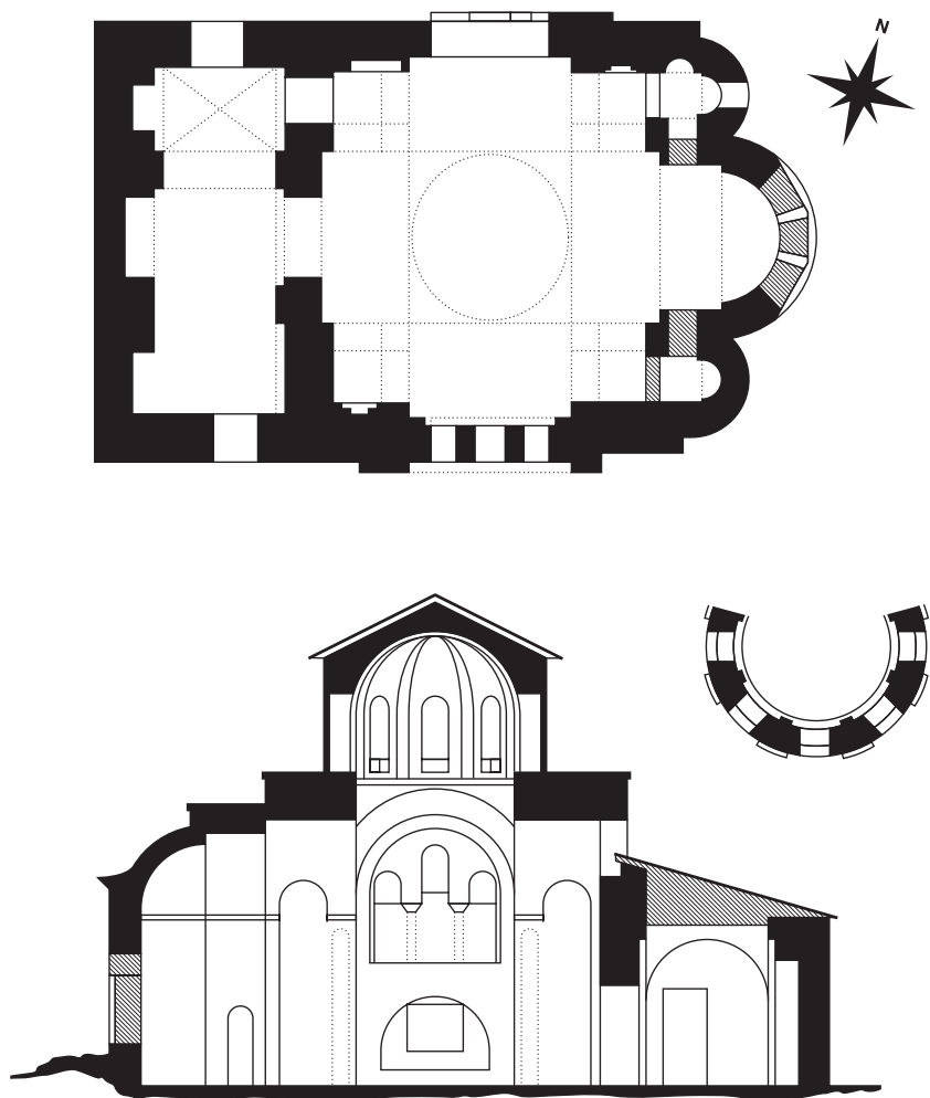
План и разрез церкви Предтечи в Трулле
