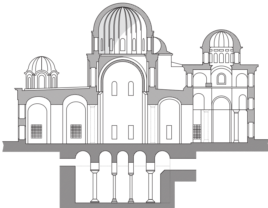
Разрез храма и цистерны Паммакаристос
