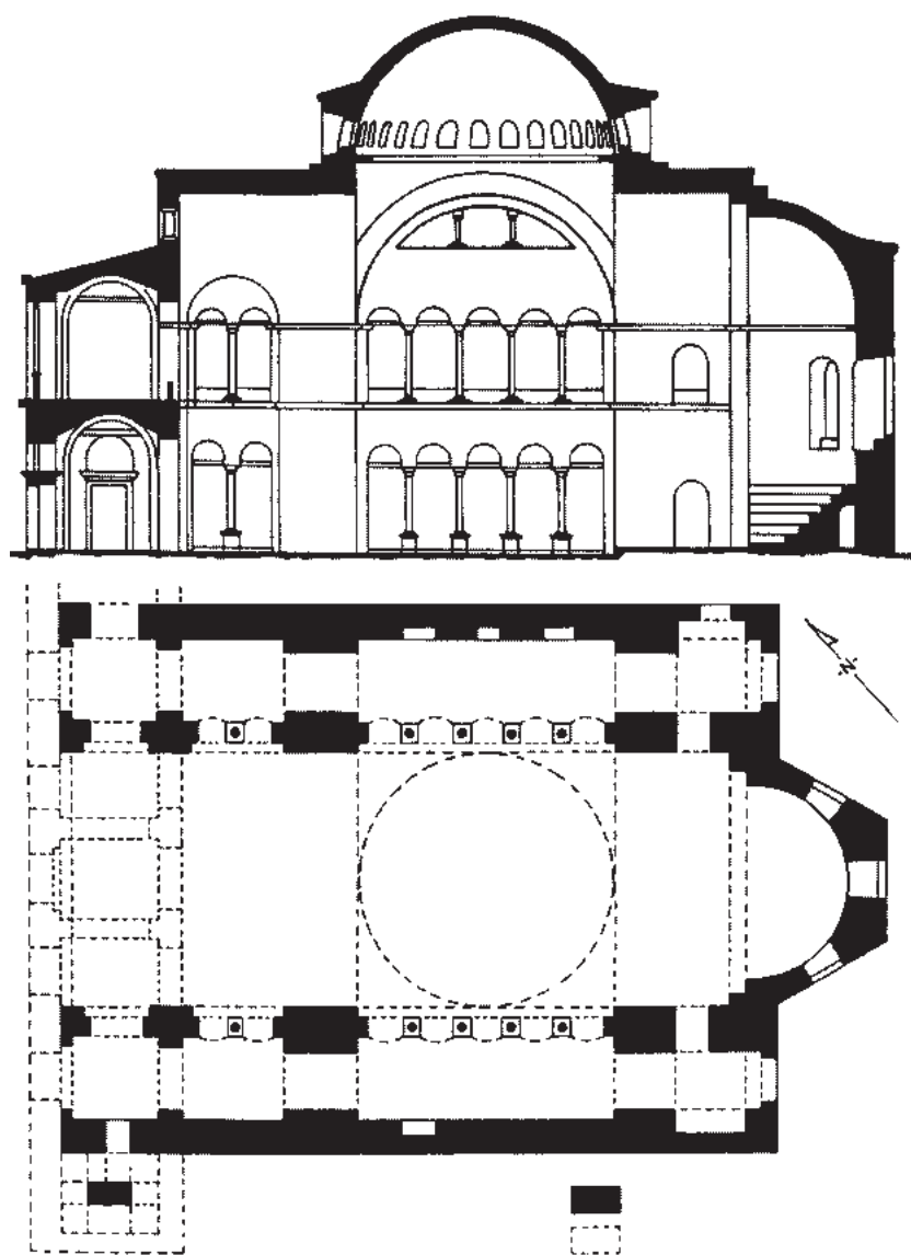
Продольный разрез и план храма Св. Ирины
