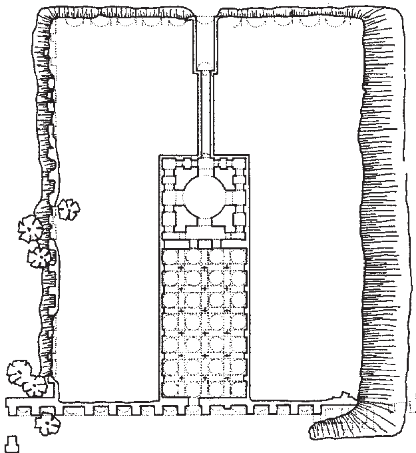
Цистерна монастыря Сатира
