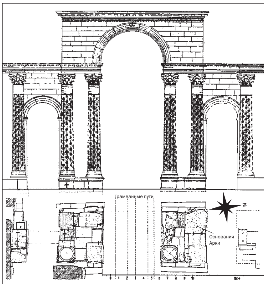
Реконструкция и план арки Феодосия
