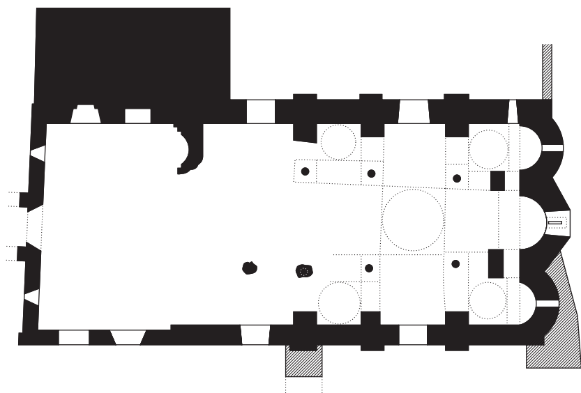
План византийской церкви Панагии Пантовасилиссы
