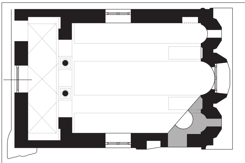
План византийской церкви Manastir Mescidi
