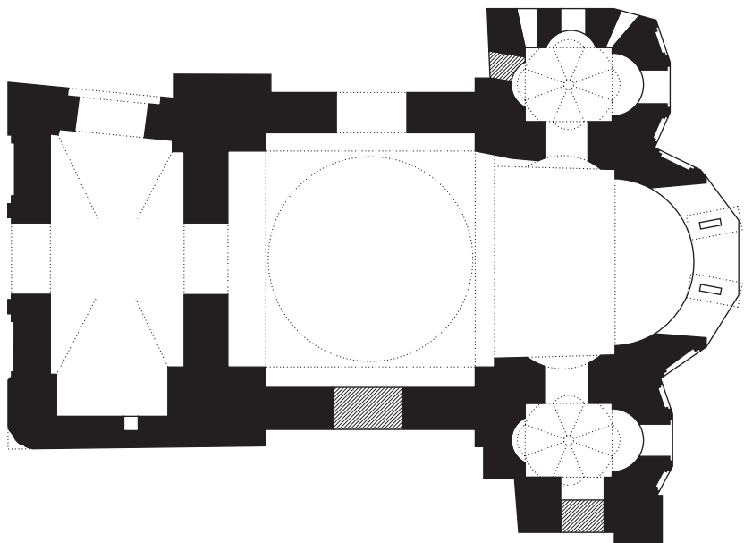
План церкви Св. Аверкия
