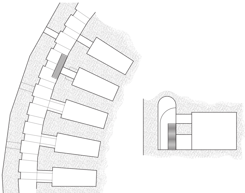
Сфендона в плане и в разрезе
