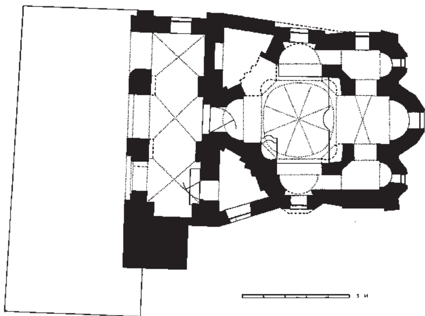
План церкви Панагии Камариотиссы
