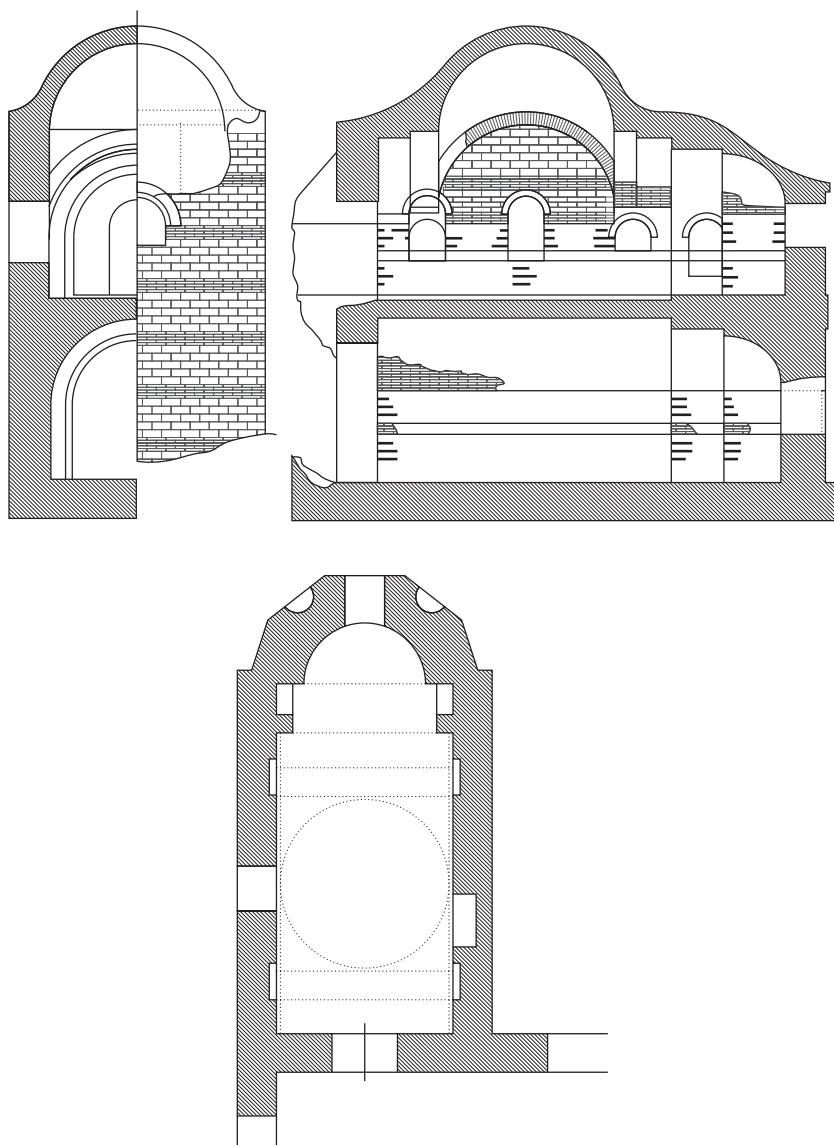
Разрез и план Bogdan Sarayı
