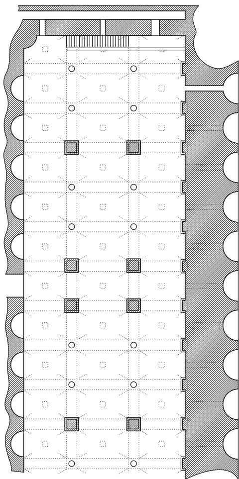
План и разрез цистерны на бульваре Ататюрка
