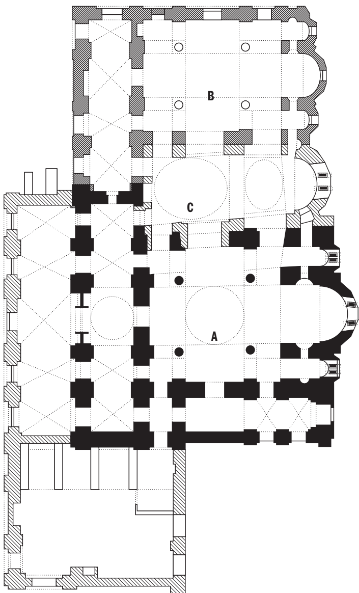
План церкви Пантократора
